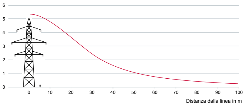
Intensità del campo magnetico a livello del suolo in microtesla (linea in esercizio a pieno carico a 2240 A)
